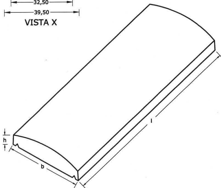
ASSONOMETRIA
